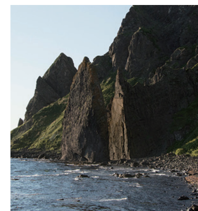
9 地藏岩 元地海岸にそび え立つ、お地藏様 が手を合わせて 拝んでいるように 見える巨岩。
