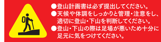
標高差 1,490m 登り約6時間、下り約4時間
